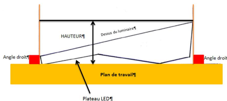
Vue de côté du luminaire
