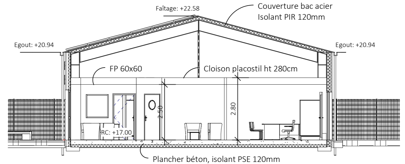
COUPE CC' Ech : 1 : 100
