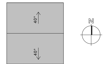
Plan de toitures Ech: 1/200
