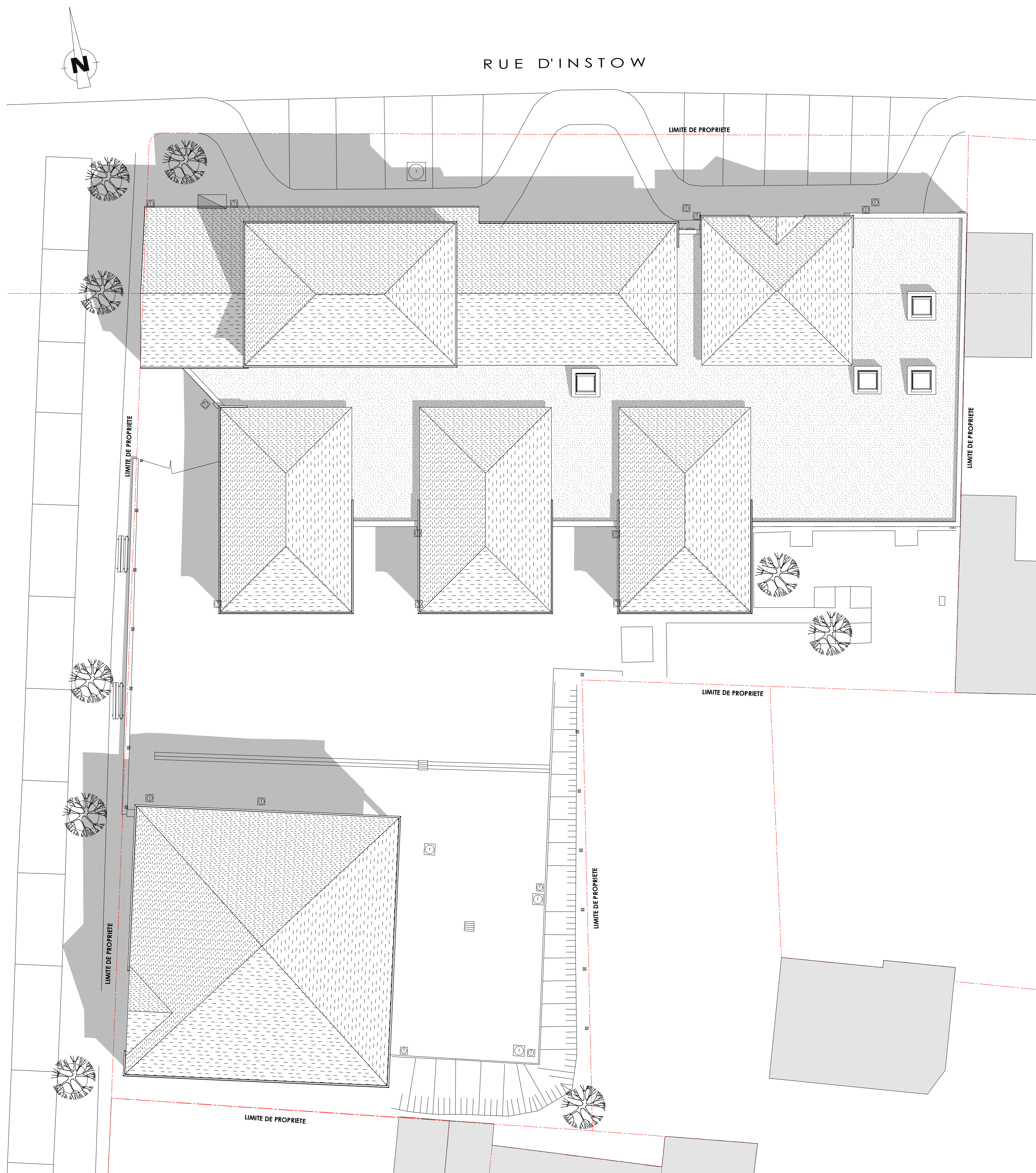
PLAN DE TOITURE EXISTANT - ECH : 1/100
