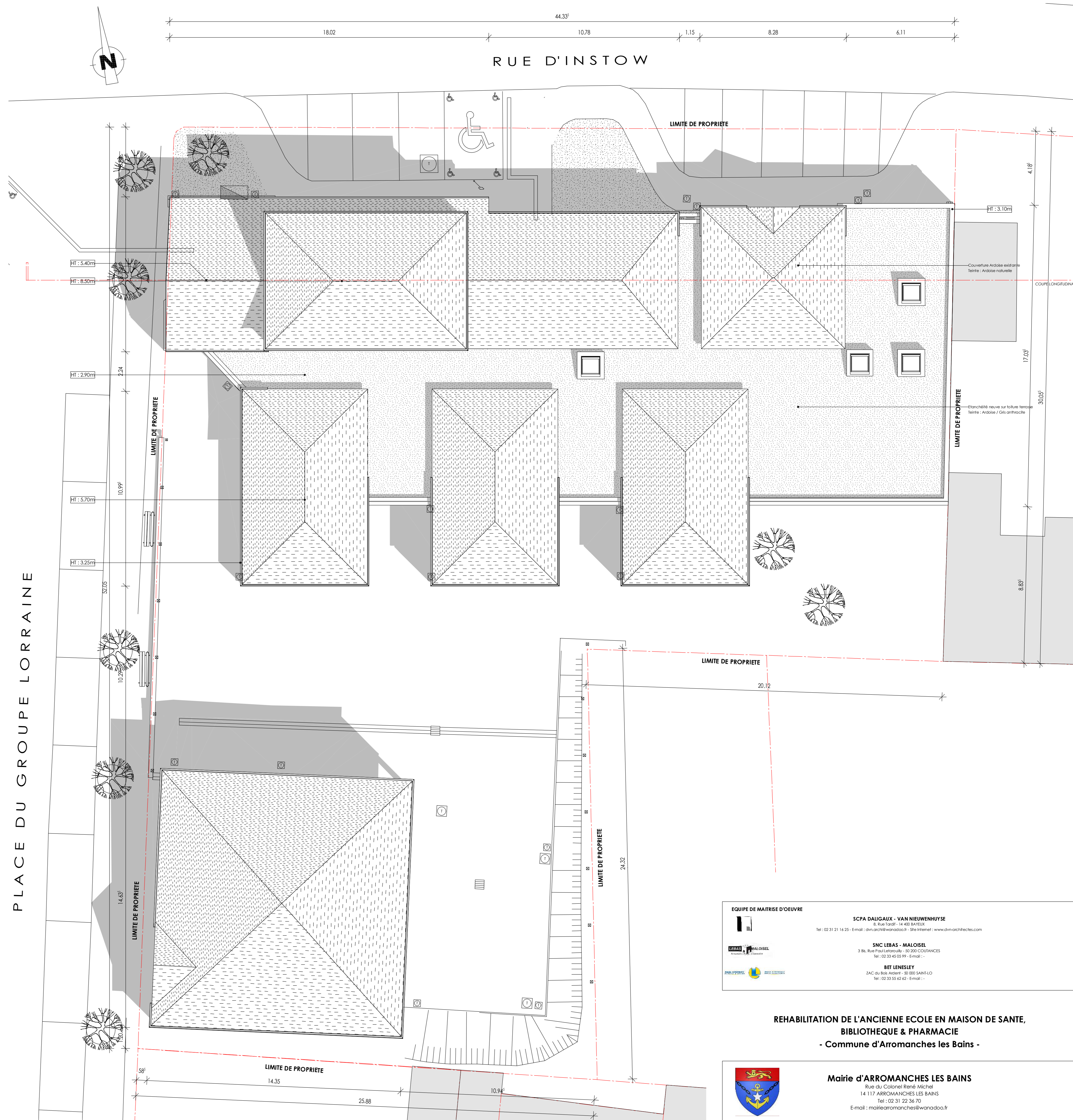
PLAN DE TOITURE PROJET - ECH : 1/100
